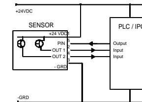
Abb.4 Anschlussbeispiel für digitale Sensoren mit Blechdicken-Teach-in Programmierung und Doppelblechschaltausgang
