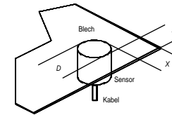
Abb.3 Sensorposition zum Blechrand, beidseitige Sensoren:
