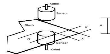
Abb.4 Anschlussbeispiel für digitale Sensoren mit Blechdicken-Teach-in Programmierung und Doppelblechschaltausgang
